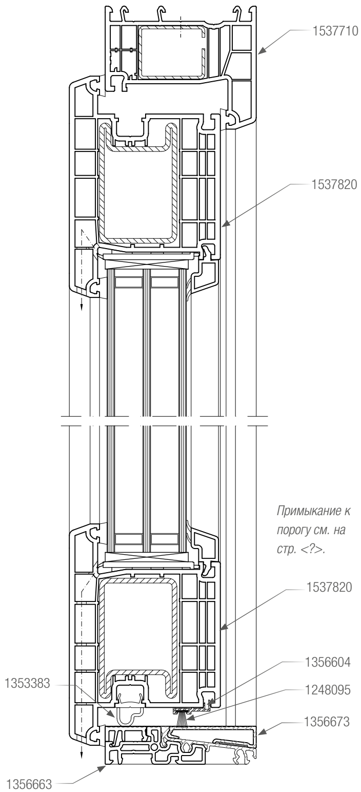
A - A
